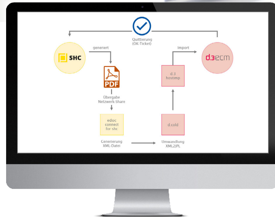
Abb.: Asynchrone Archivierung mittels Serverprozessen
